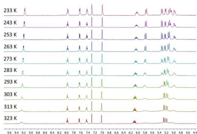
Fig. 6 VT ^1\text{H} NMR spectra (500 MHz, \text{CD}_3\text{CN} ) of complex 7e (233 – 323 K).
