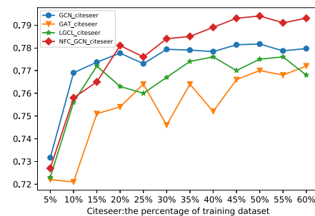
(b) Citeseer
