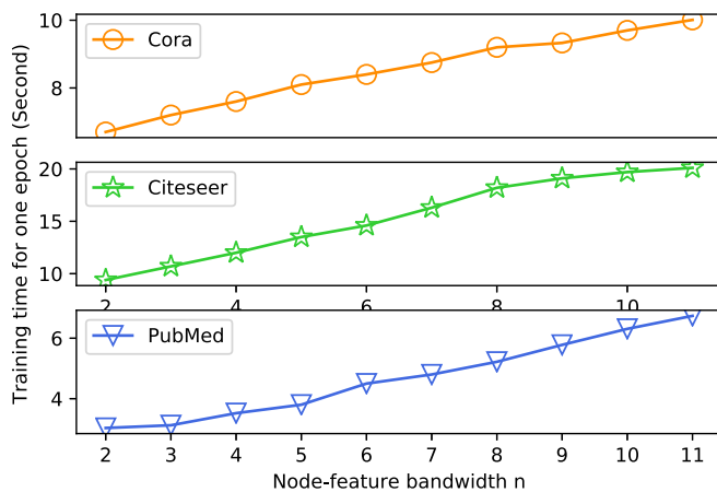
(b) Time per epoch.
