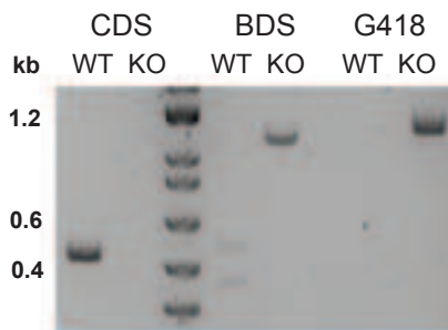
LmCALP25.1 (LmxM.25.1480)
