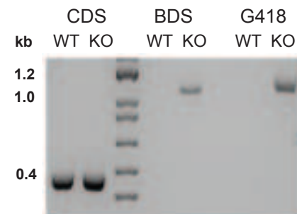
LmCALP31.6 (LmxM.30.0460a)
