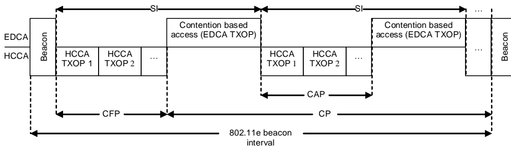
Fig. 1. The 802.11e superframe
