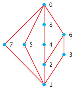
Fig. 2. The lattice (0 \dots 8, \text{divides}) .
