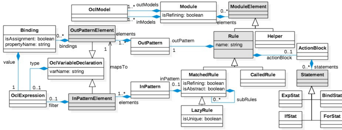
Fig. 2. ATL metamodel
