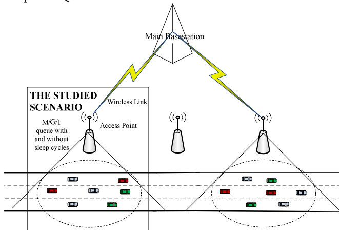
Fig. 1: Motorway Scenario.
