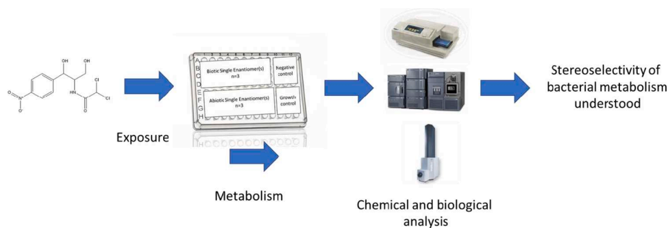
Fig. 3. SAM workflow
