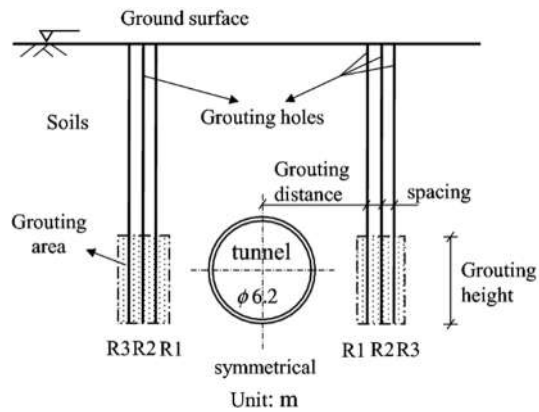
Fig. 40. Grouting parameters layout [177].
