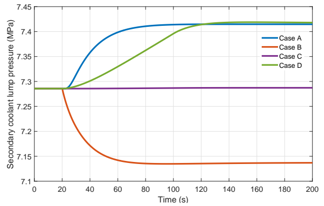
(d) Steam generator pressure.
