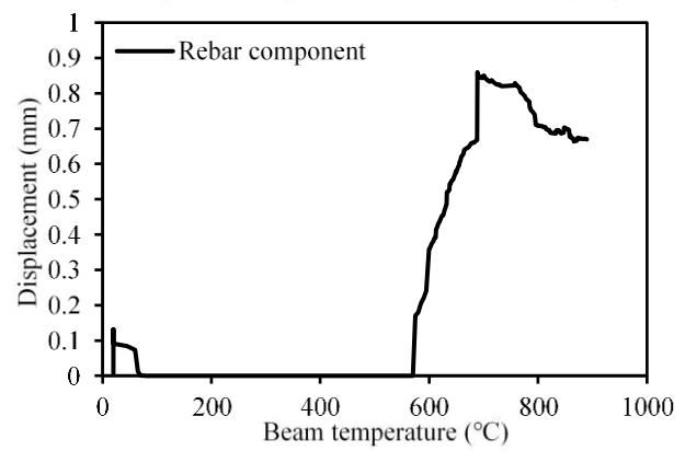
(d) Temperature-displacement curve of rebar component
