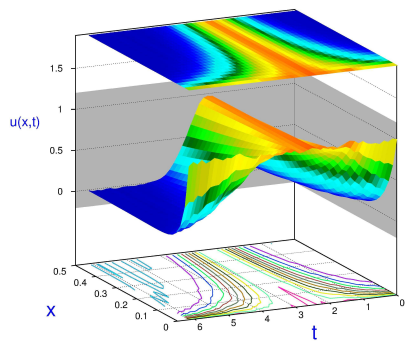
(d) u^\varepsilon(x, t), \gamma(\varepsilon) = 10^{-3}
