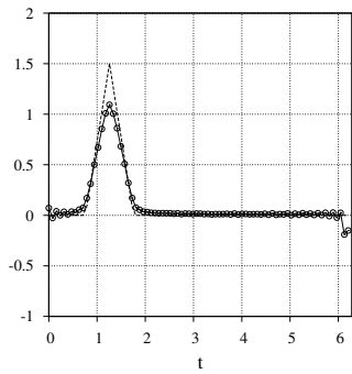
(d) \varepsilon = 2 \times 10^{-3} , \gamma(\varepsilon) = 10^{-1} .
